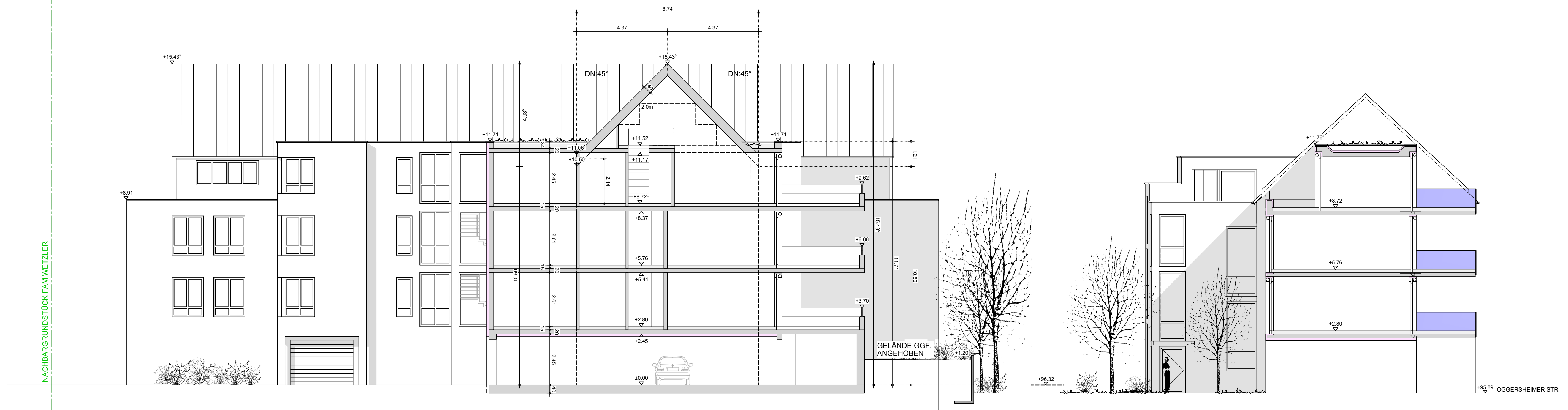
ANSICHT NORDEN 1:100
